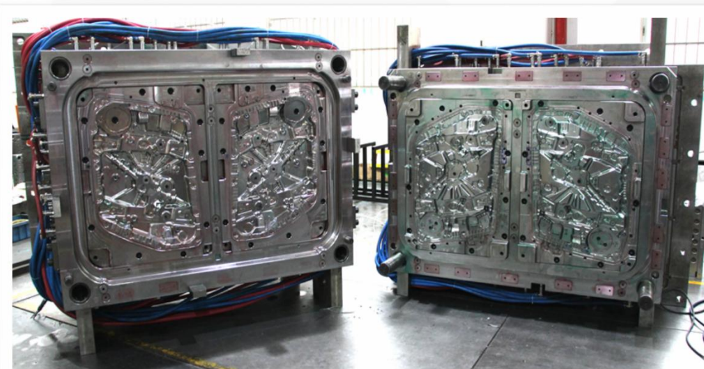
Auto Part - Door Panel
